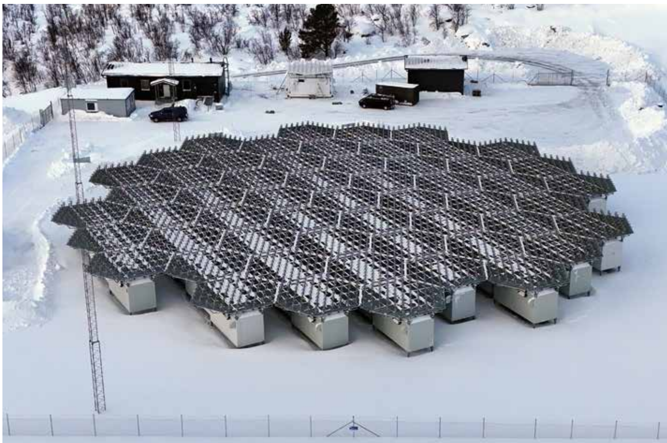
Bild 3.22: Det nya radarsystemet EISCAT_3D är tänkt att resultera i mätningar med flerfaldigt högre rums- och tidsupplösning och samtidiga observationer över stora volymer. Radarsystemet kommer att användas frekvent av forskare vid IRF. Bild: EISCAT
